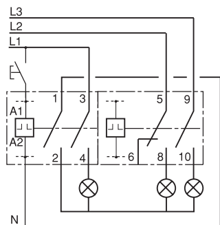
Импульсное реле TL 16 A с ETL, 3 полюса + нейтраль
