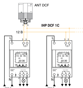
К одной антенне подключаются до 5 IHP DCF
