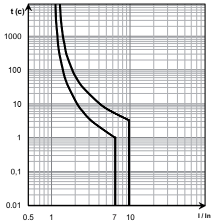
С60Н-ДС, кривая С
