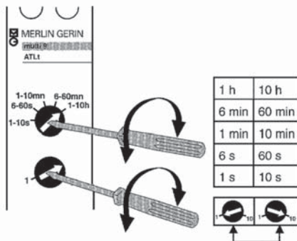
Настройка таймера ATLt
