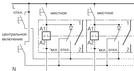
Импульсное реле ТЛс
