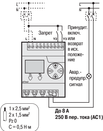
Запрет / Принудительное включение / Аварийно-предупредительная сигнализация
