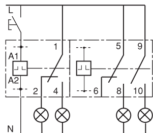
Импульсное реле TL 16 A с ETL
