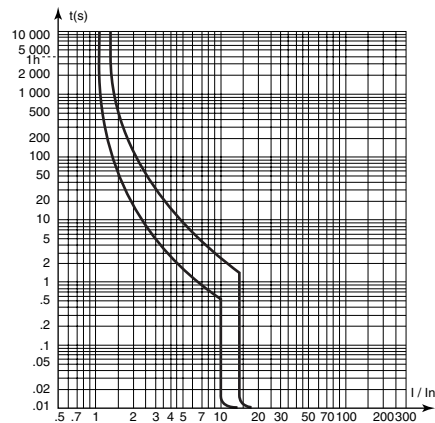
С60Н-ДС, кривая С
